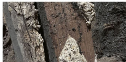
Hausschwammbefall Kirche Niedersteinbach Fotos: Johannes Möller
